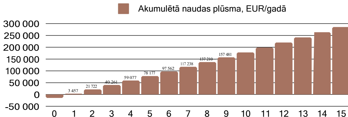
71. attēls. Neto naudas plūsma un akumulētā naudas plūsma
