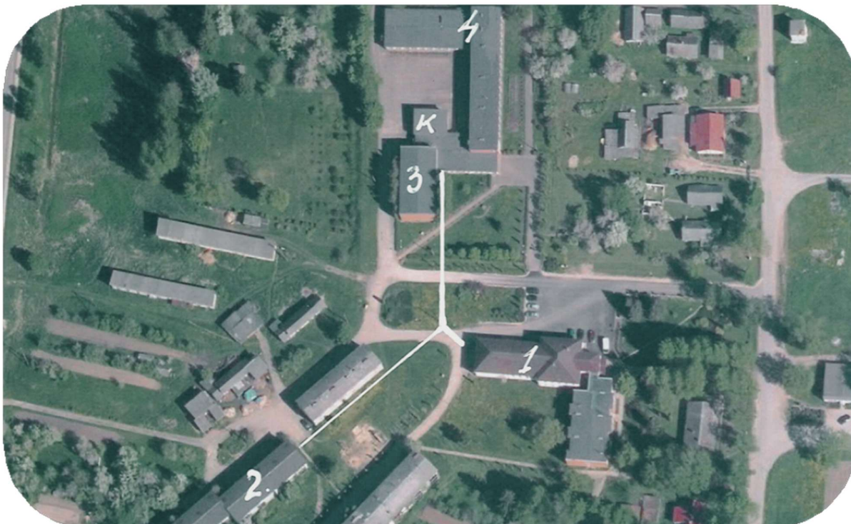
74. attēls. Katlumājas lokācija, apkurināmās ēkas un siltumtrase
