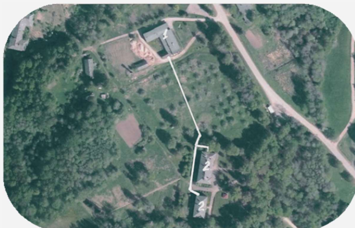
64. attēls. Katlumājas lokācija, apkurināmās ēkas un siltumtrase
