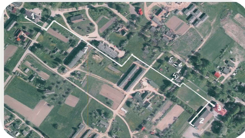
54. attēls. Katlumājas lokācija, apkurināmās ēkas un siltumtrase
